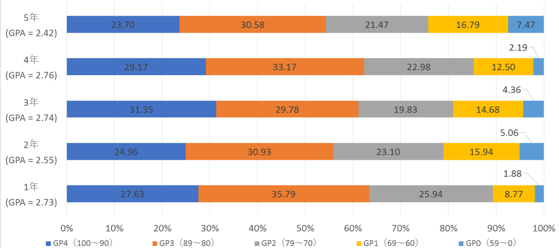
2021年度本科学年ごとのGPの分布
